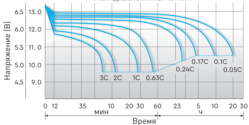
РАЗРЯДНЫЕ ХАРАКТЕРИСТИКИ
