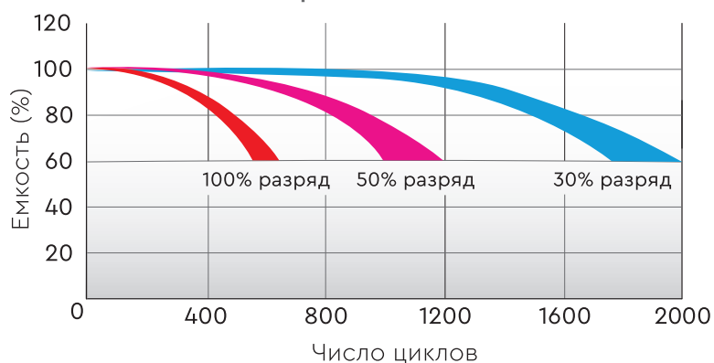
СРОК СЛУЖБЫ В ЦИКЛИЧЕСКОМ РЕЖИМЕ (до 55 Ач)
