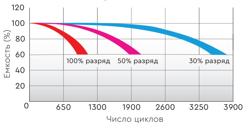
СРОК СЛУЖБЫ В ЦИКЛИЧЕСКОМ РЕЖИМЕ (от 100 Ач)
